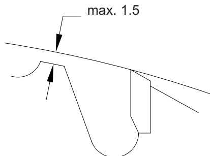
AKE Chip Limiter Limiteur de copeaux AKE
